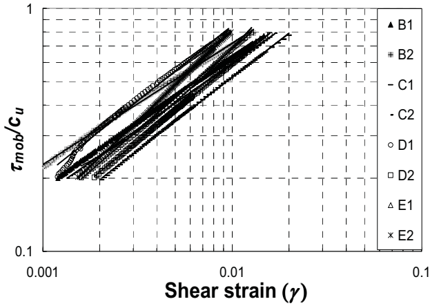
a) Yimsiri (2001)
