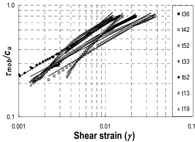
b) Gasparre (2005)
